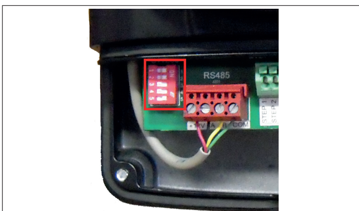
Position der Schalter zur Steuerung über die Benutzerschnittstelle
